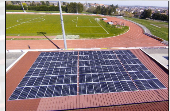
Club house Football Club de Saverne 36kWc, 200m 2 de PV
